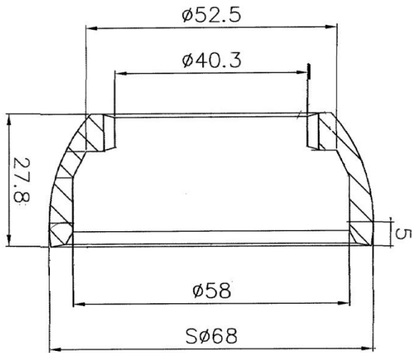
Ball Guide
